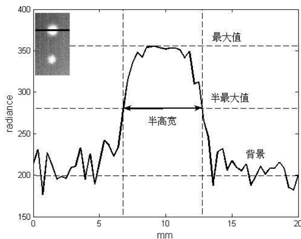
图2 缺陷中心扫描线上的辐射量分布
